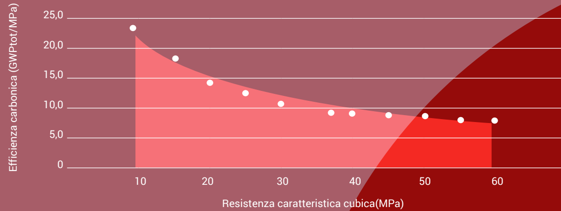
Grafico 1: curva dell'efficienza dei calcestruzzi di riferimento (senza obiettivi di sostenibilità)
